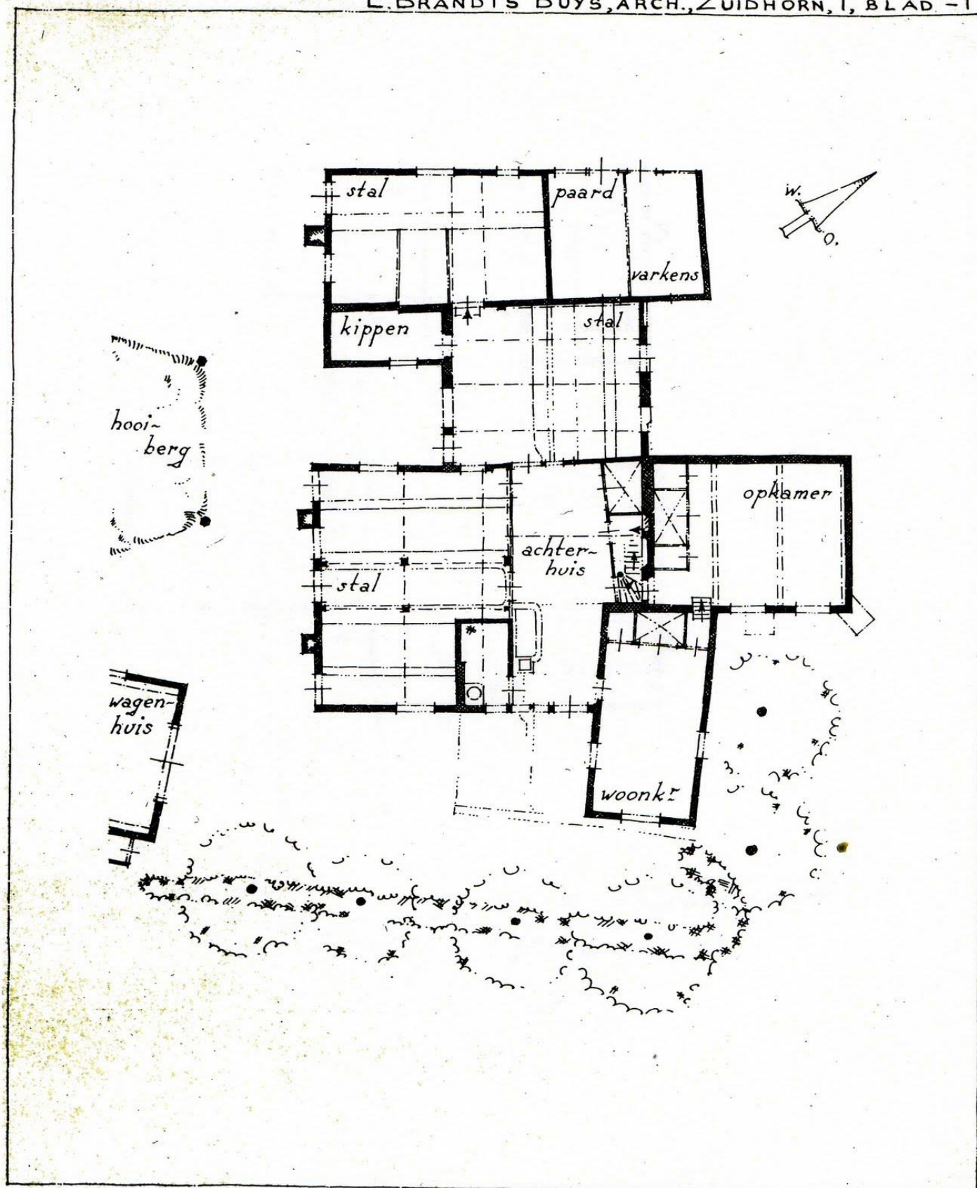
Plattegrond boerderij De Witte Raaf in Noordwijk, opgemeten en getekend door architect L. Brandts Buys (Zuidhorn), zonder jaartal
